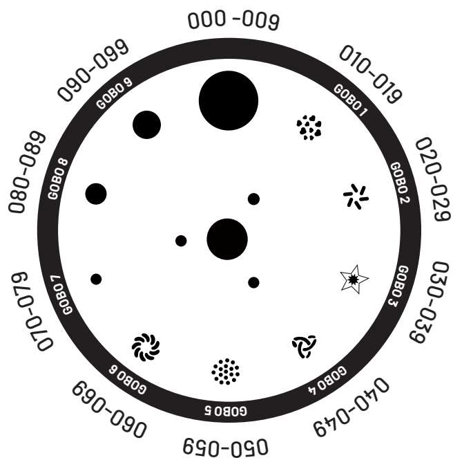
RUEDA DE GOBOS FIJOS
